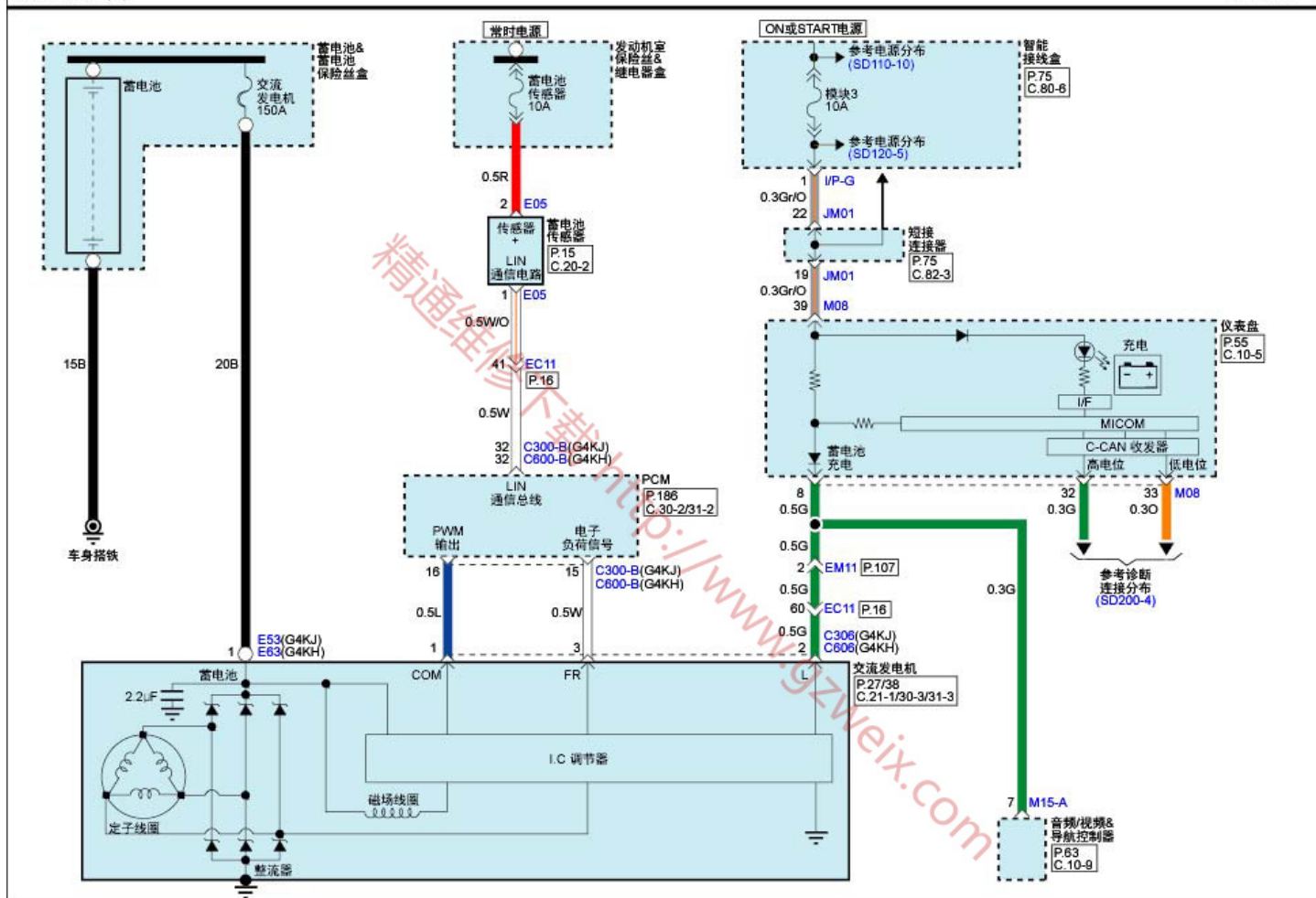
充电系统(1)
